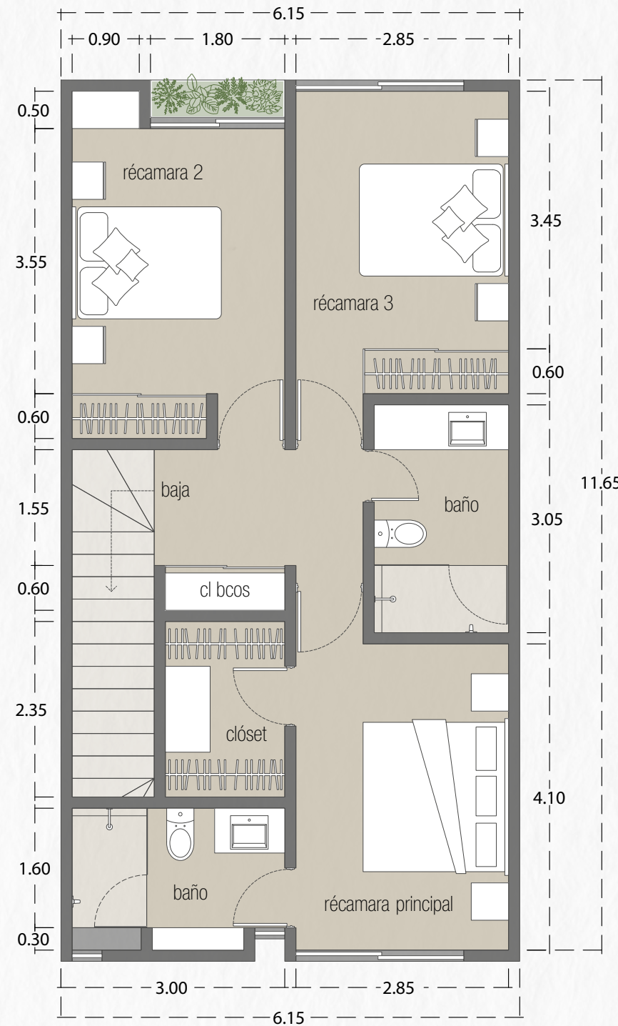
PLANTA ALTA (EN NIVEL 1)
