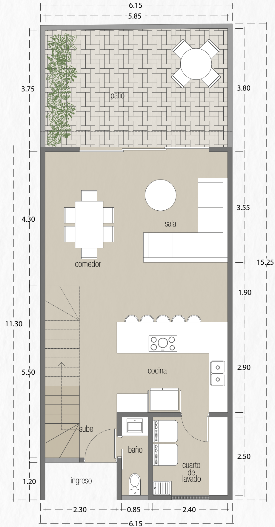
PLANTA BAJA (EN NIVEL PB)
