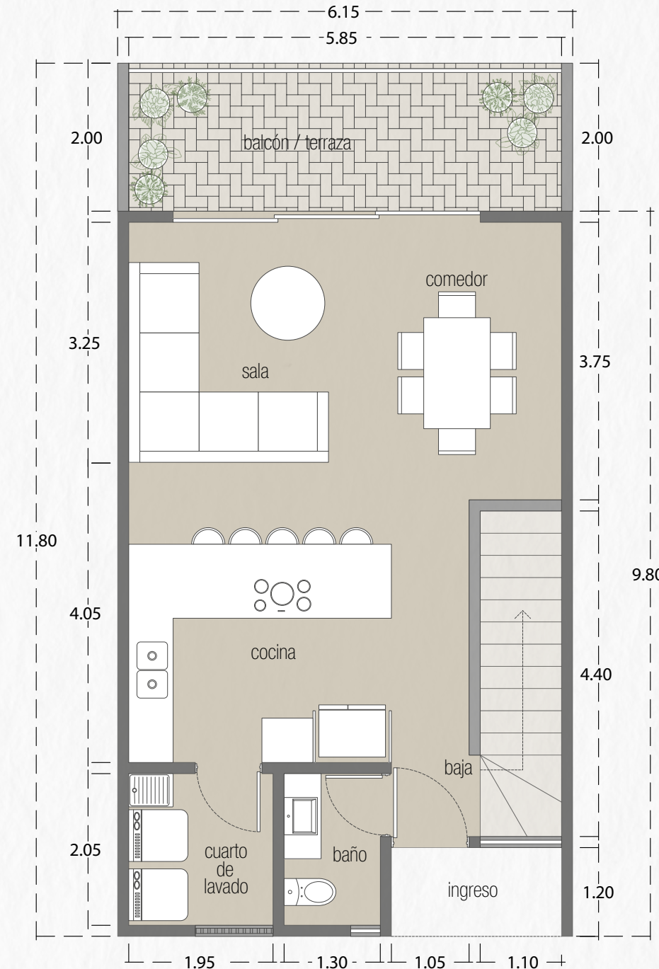
PLANTA ALTA (EN NIVEL 3)
