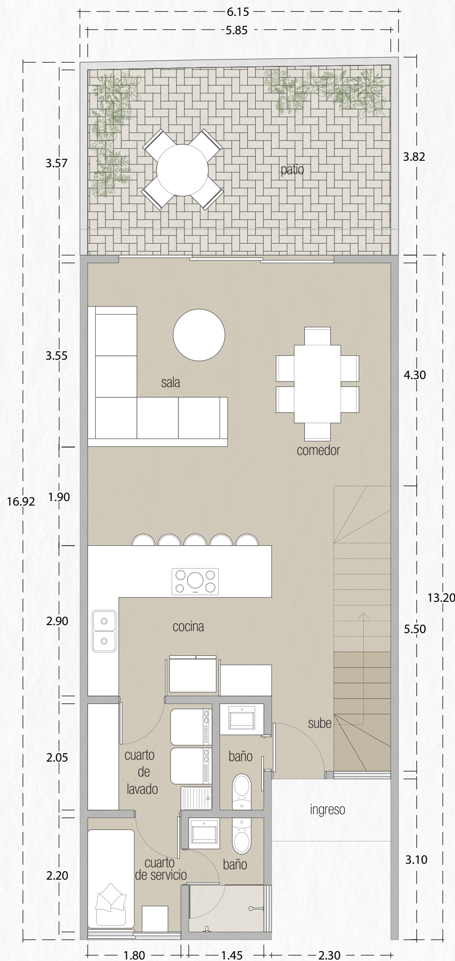
PLANTA BAJA (EN NIVEL PB)
