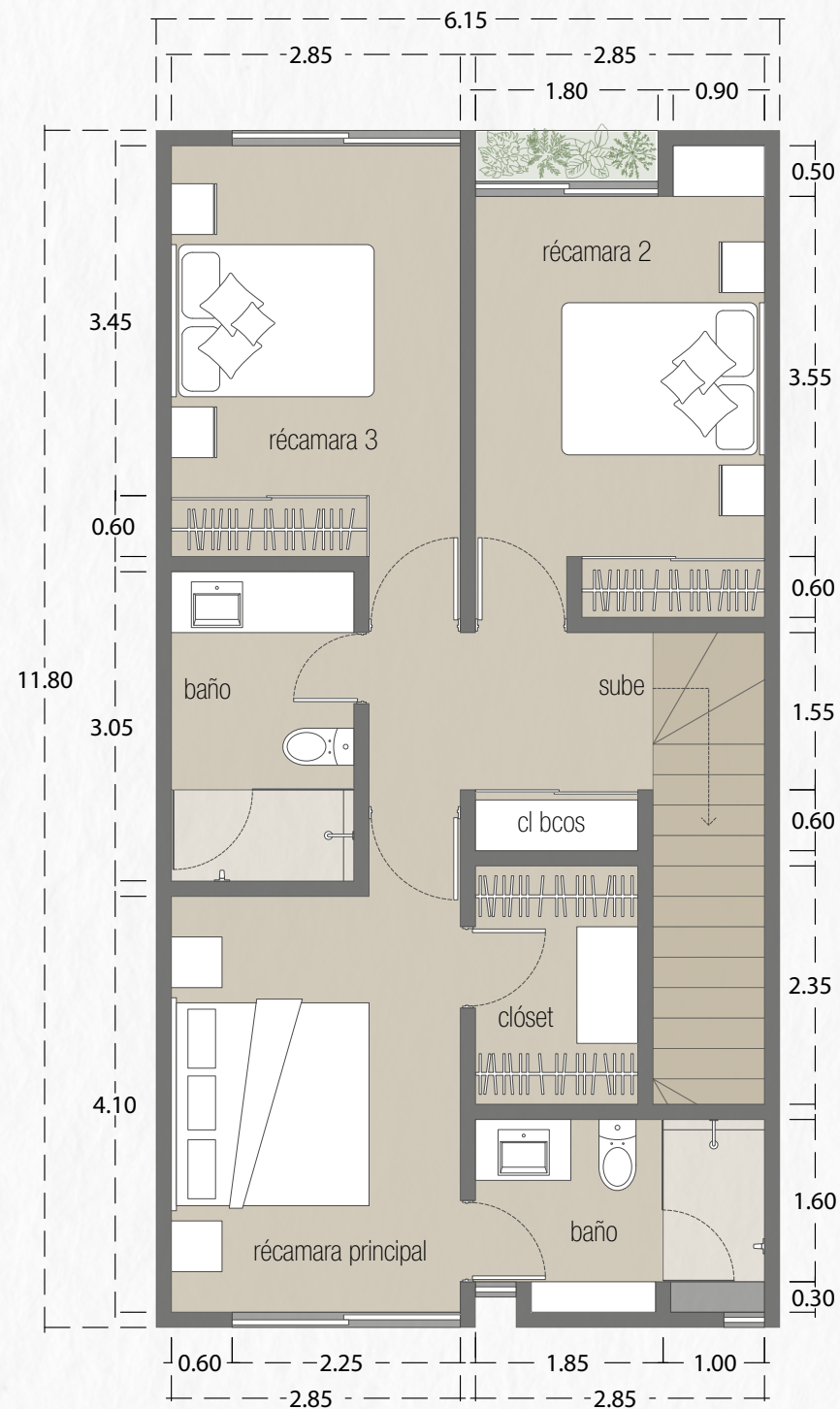
PLANTA BAJA (EN NIVEL 2)
