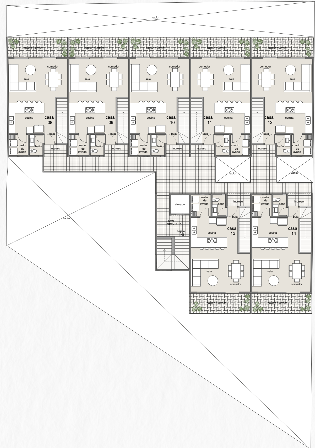
PLANTA NIVEL 3 7 CASAS (INGRESO), NÚCLEO DE ESCALERAS Y ELEVADOR.
